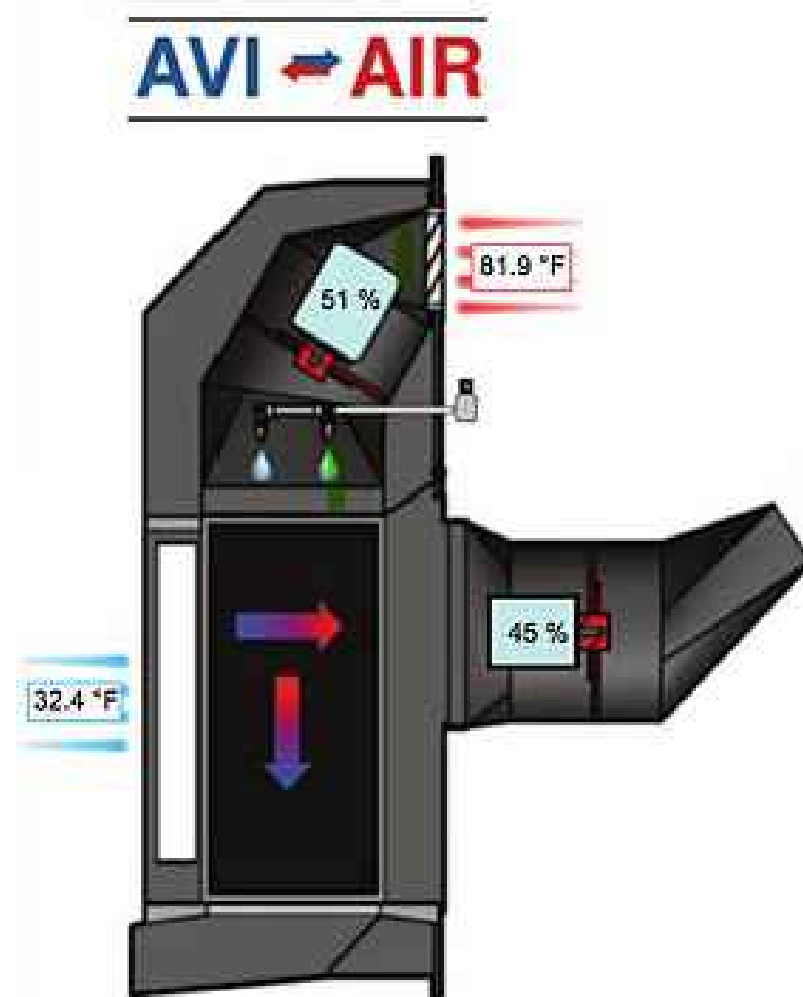
Échangeur de chaleur
